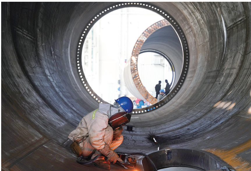
10月23日，昌吉州泰胜风能风电设备有限公司生产车间，工人正忙着生产风机塔筒。 □本报记者 常谊谊摄
